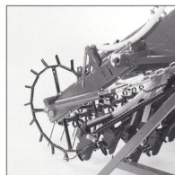
Drivhjul innanför arbetsbredden. Alltid samma arbetsförhållanden.
