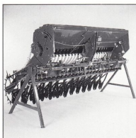
Fördelaktig infästning i förhållande till tyngdpunkten. Stödben
