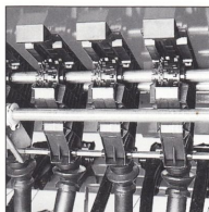
Kombimatarvals för sådd av både stora och små frön
